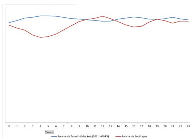
Moyenne horaire des transits 2 et soutirages sur le réseau HTB3, 2011
