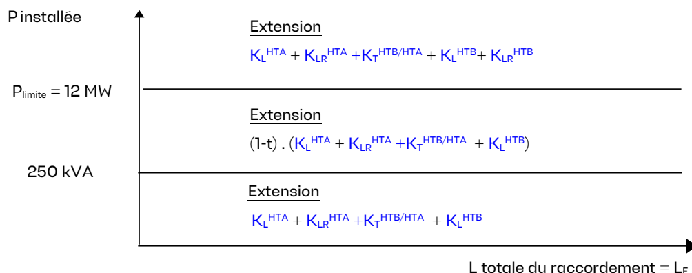
Figure 7 : composants de la facturation des extensions en HTA
