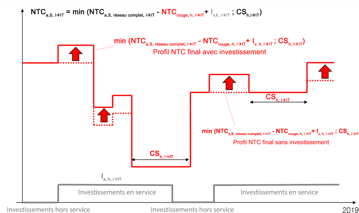
Schéma 11 : Calcul du profil horaire de la NTC finale en prenant en compte l'inclusion générale d'un nouvel investissement de réseau et son profil de valeur d'investissement horaire (selon son programme de disponibilité).
