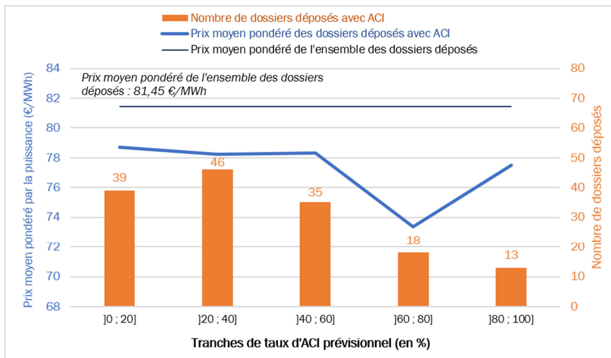
Figure 7 – Prix moyen pondéré par la puissance en fonction des tranches de taux d'ACI prévisionnel pour les installations ayant déclaré participer à une opération d'ACI
