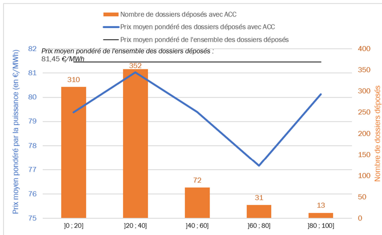
Figure 8 – Prix moyen pondéré par la puissance en fonction des tranches de taux d'ACC prévisionnel pour les installations ayant déclaré participer à une opération d'autoconsommation collective
