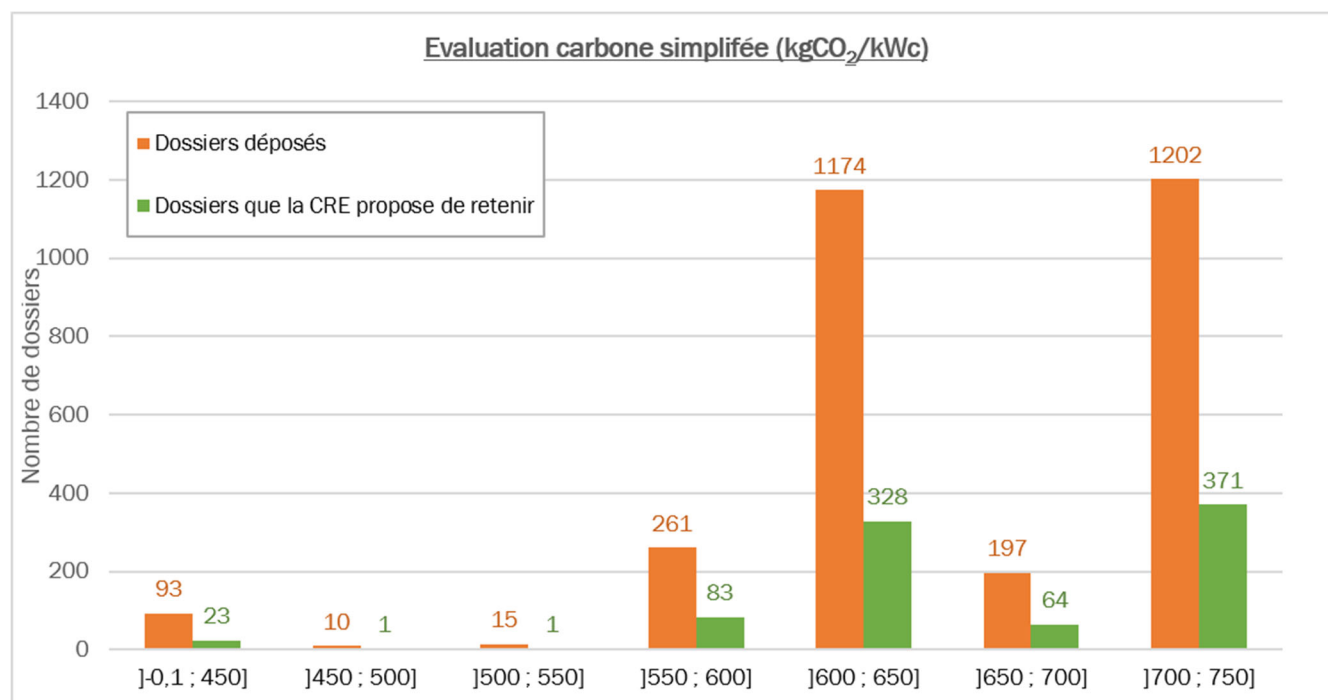
Figure 6 – Répartition des dossiers par tranche de valeur d'ECS pour les modules photovoltaïques
